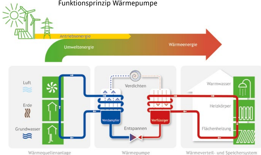
Funktionsprinzip Wärmepumpe
