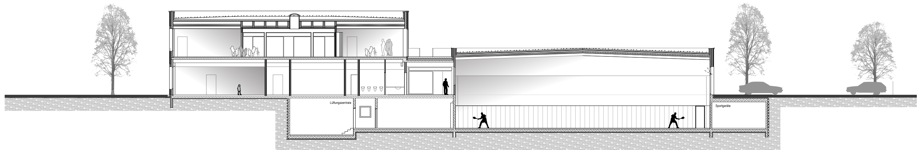
Querschnitt Schule/Sporthalle
