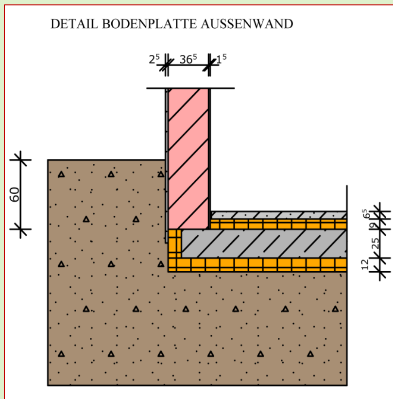
Anschluss Bodenplatte – Außenwand
