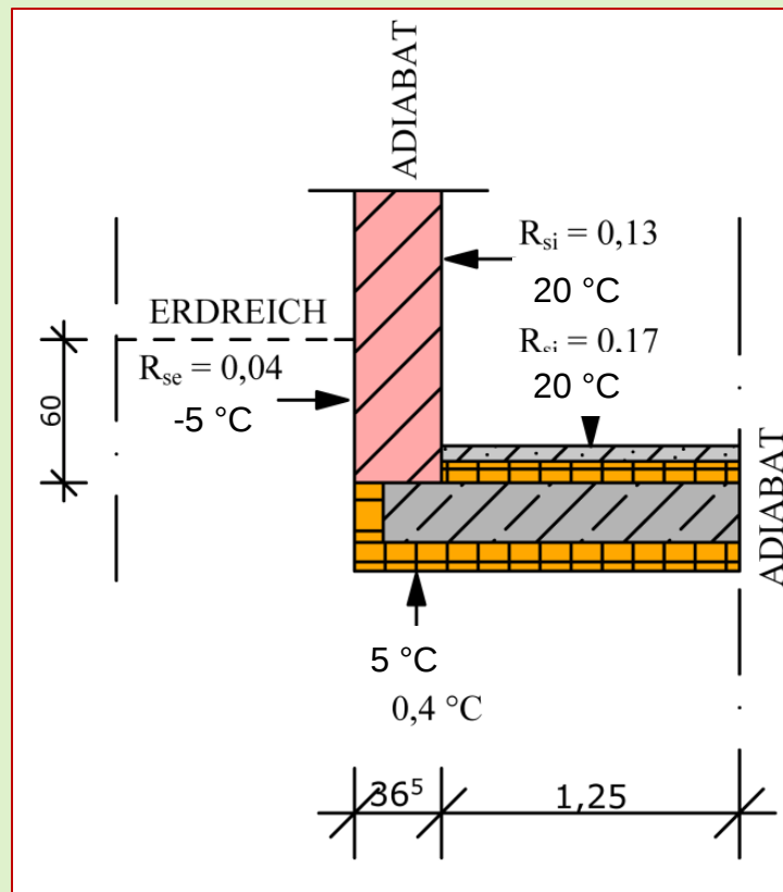
Darstellung der Randbedingungen für die Berechnung des Sockeldetails – Erdreichanschüttung \leq 1\text{m}
