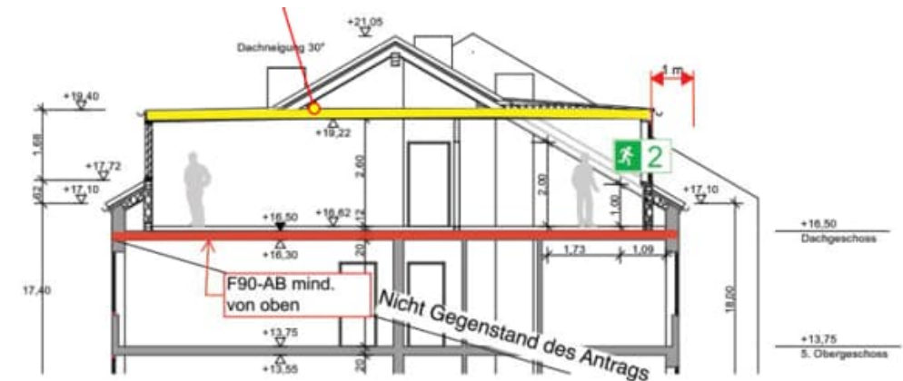
Schnitt B
