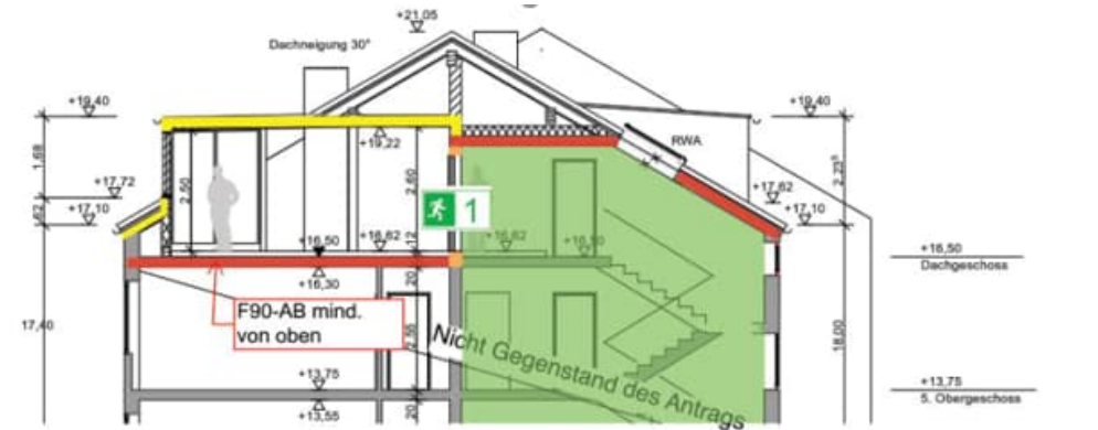
Schnitt A
