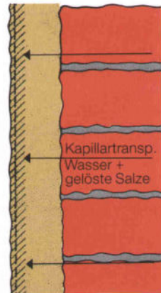
Verdunstungszone
