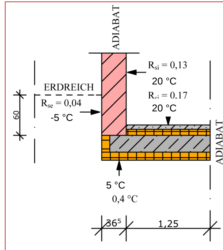
Darstellung der Randbedingungen für die Berechnung des Sockeldetails – Erdreichanschüttung \leq 1\text{m}
