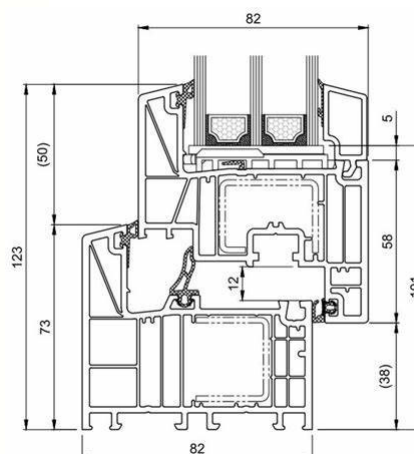
Mitteldichtungssystem
