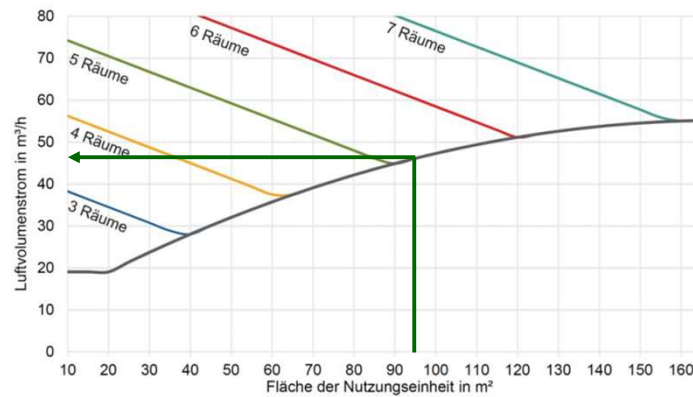
Bild B.1 Notwendiger Volumenstrom über alle Fensterlüfter für Lüftung zum Feuchteschutz in Abhängigkeit der Fläche der Nutzungseinheit und der Anzahl der Räume: • eingeschossige Nutzungseinheit, Etagenwohnung im Mehrfamilienhaus • geringer Wärmeschutz, nicht modernisiert oder nur Teilmodernisierung • windschwacher Gebäudestandort • hohe Belegung (< 40 m²/Person)
