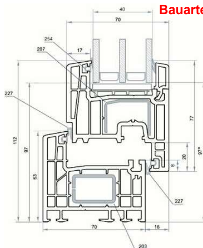
Anschlagdichtungssystem
